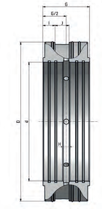
ROTODISK SW 65-150
