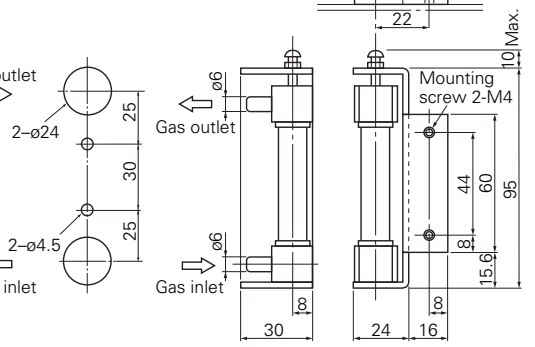
Panel cutout (ZBD5)
