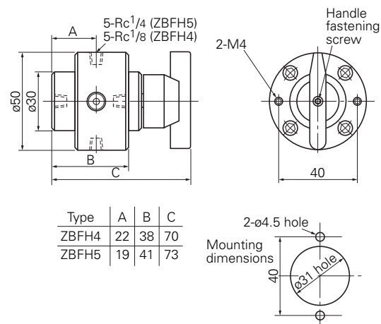
4-way valve (ZBFH4/ZBFH5)
