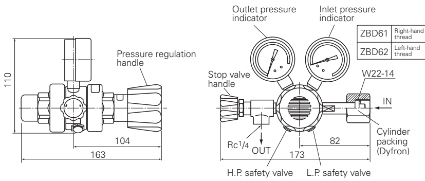
Pressure regulator (ZBD61/ZBD62)
