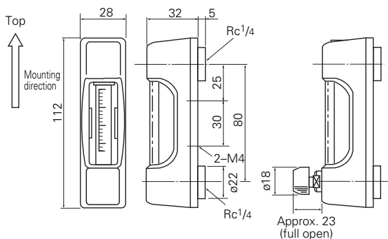
Flow meter (ZBD57)
