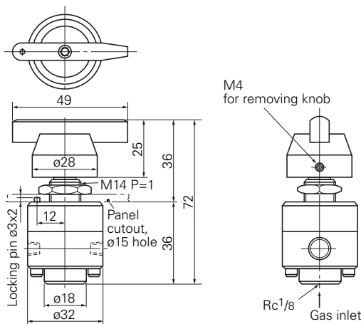
2-way valve (ZBFH2)
