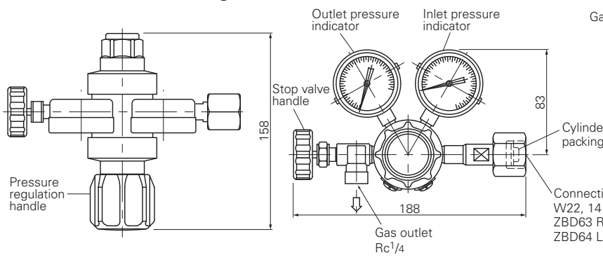
Pressure regulator (ZBD63/ZBD64)
