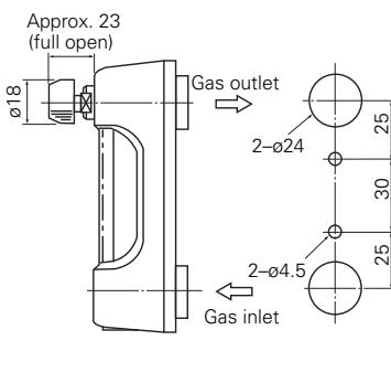
Flow meter (ZBD54)
