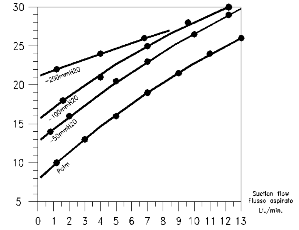
Air consumption Aria di alimentazione Lt./min.
